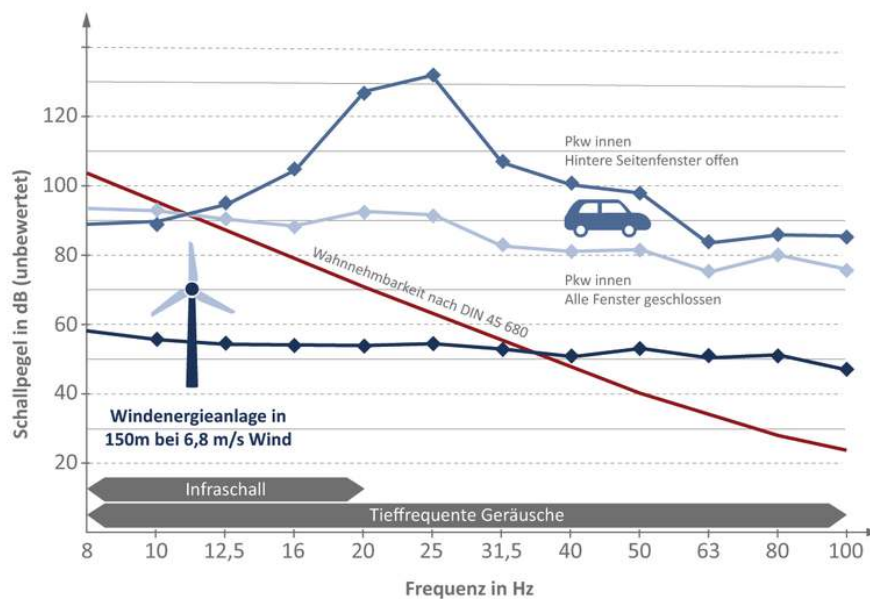
Abbildung: Infraschall und tieffrequente Geräusche von verschiedenen Emittenten
